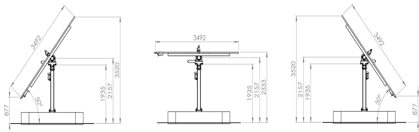
DEGER S100-CF-DR mit Betonfundament (1)
