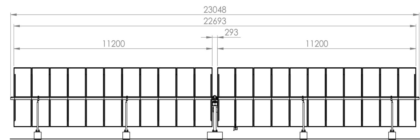
DEGER S100-CF-DR mit Betonfundament (1)
